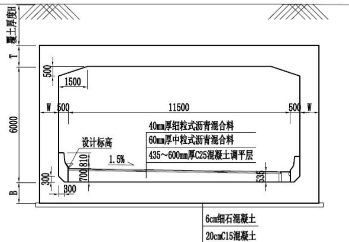
图 2-7 主线单孔净宽 12.5m 标准横断面
