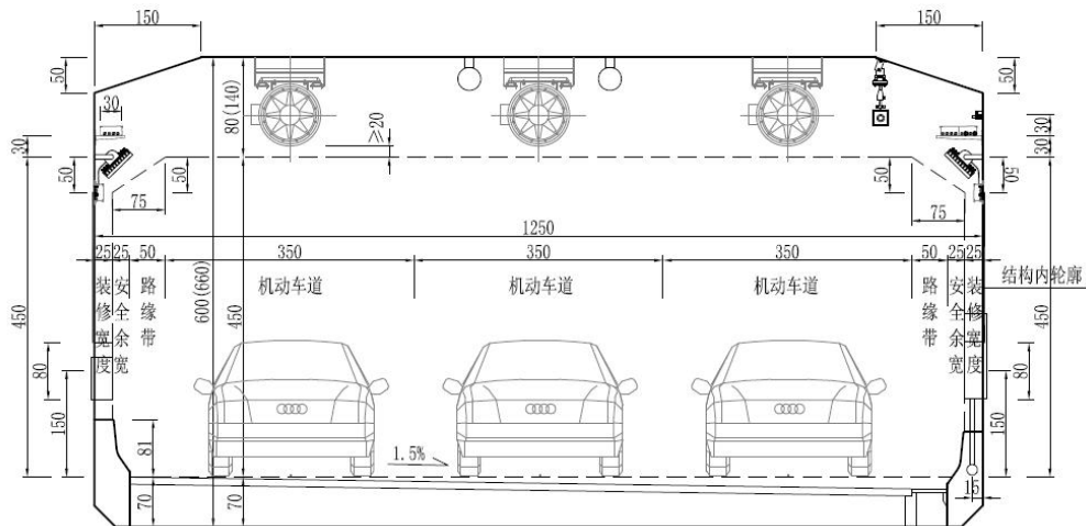
图 2-5 主线隧道建筑限界图
