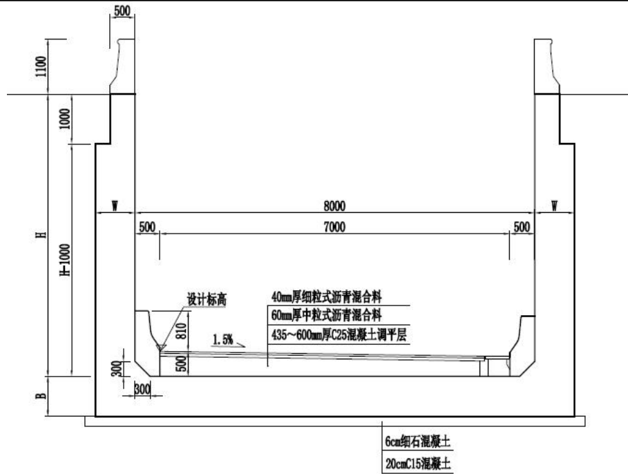
图 2-11 匝道隧道敞口段标准横断面
