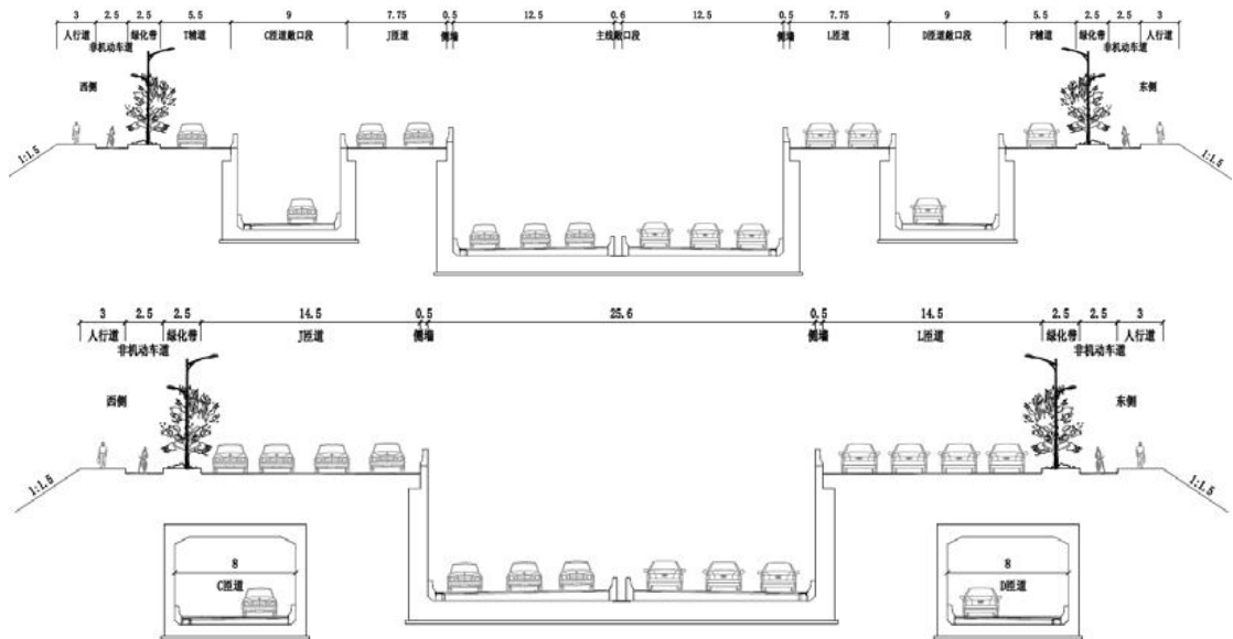
图 2-2 南湾大道以南主线道路横断面图
