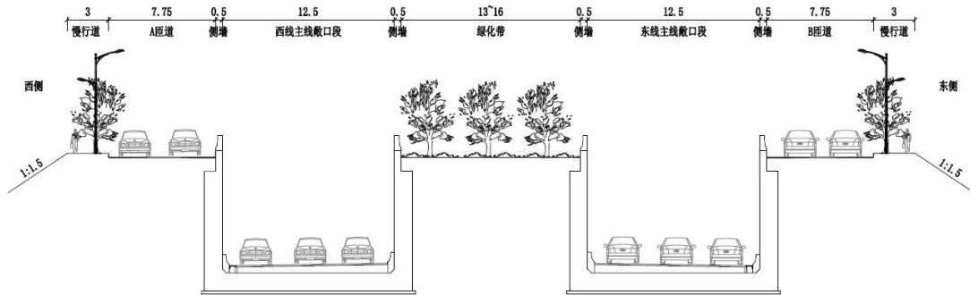
图 2-1 晨光路以北主线道路横断面图
