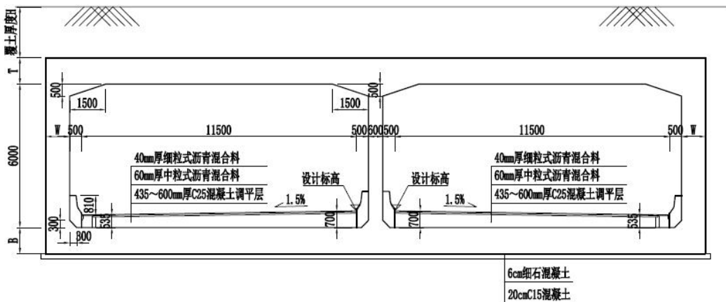
图 2-8 主线双孔净宽 2 \times 12.5\text{m} 标准横断面
