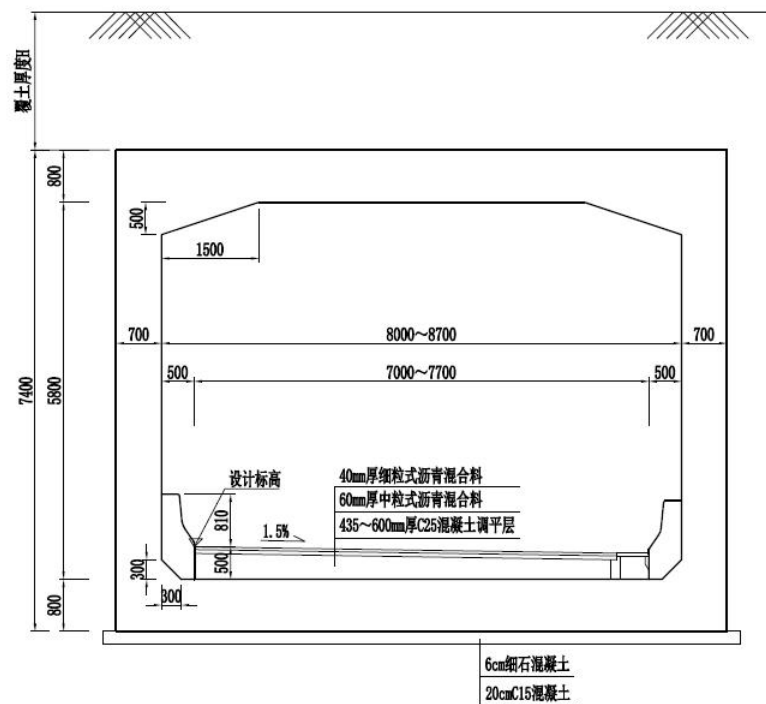
图 2-10 匝道隧道暗埋段标准横断面
