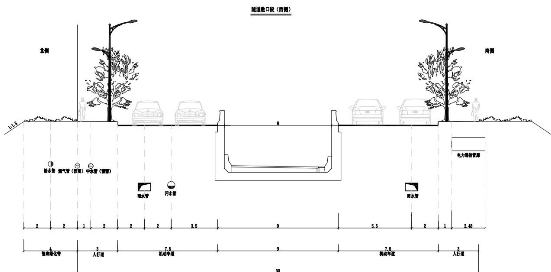
图 2-14 晨光路管线设计横断面
