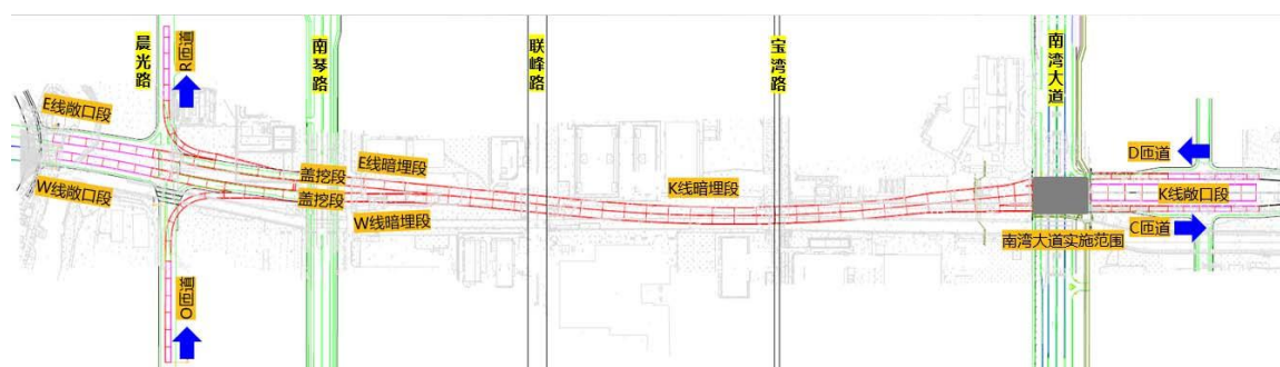
图 2-4 隧道平面布置图
