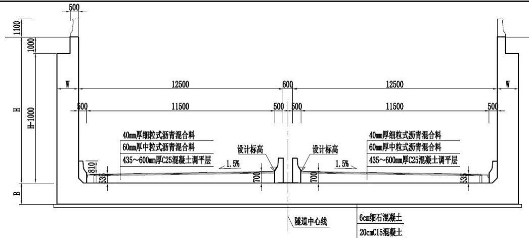
图 2-9 主线双孔净宽 2x12.5m 敞口段标准横断面
