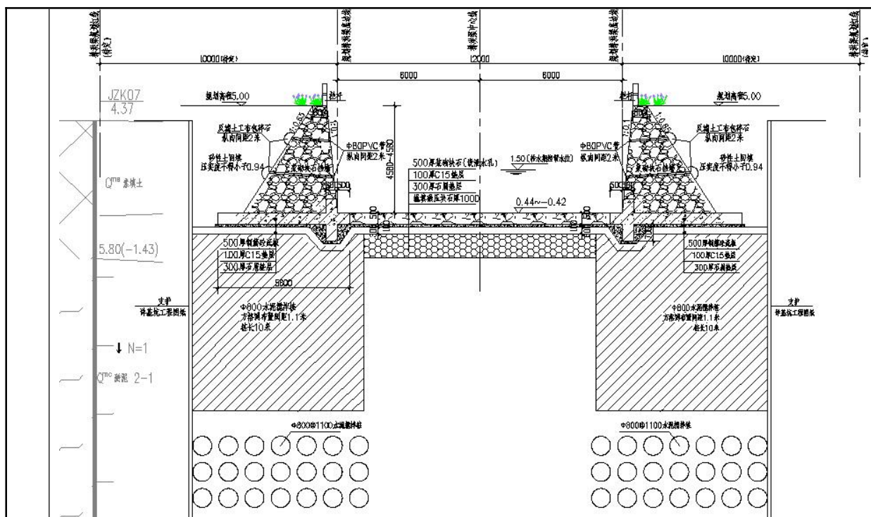
图 2-13 南琴路至保北路段、保北路~联峰路、联峰路~宝湾路、宝湾路~南湾大道排洪渠断面图
