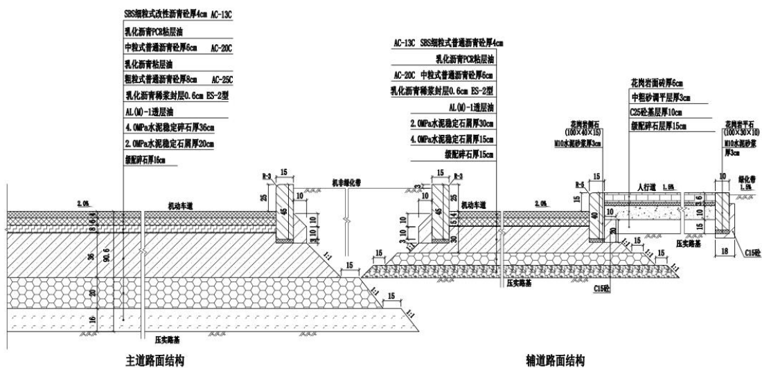
图 2-3 道路路面结构示意图
