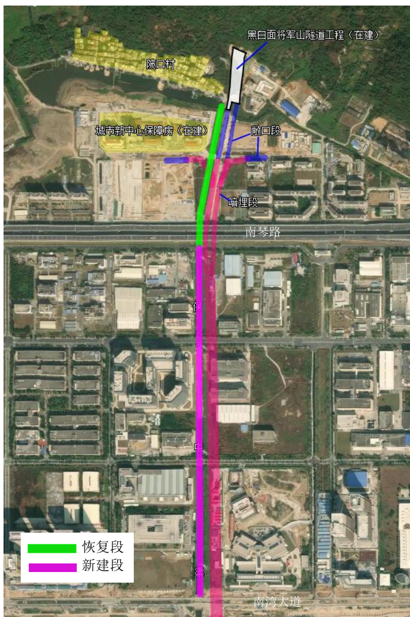
图 2-12 排洪渠工程示意图
