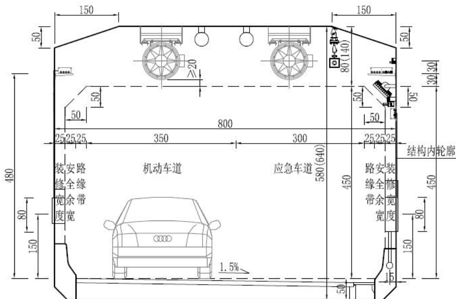
图 2-6 匝道隧道建筑限界图
